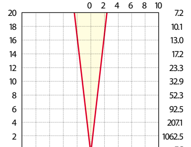
20W MR-16: LN-20 ESX
