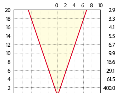
42W MR-16: LN-42 EYP
