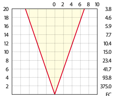
50W MR-16: LNU-50 EXN
